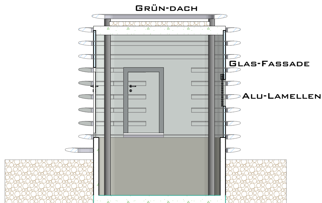
SCHNITT
