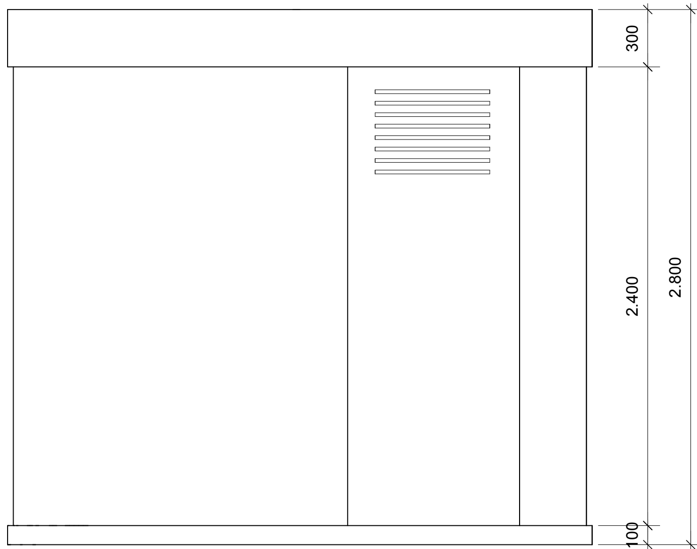
Ansicht 1:20
