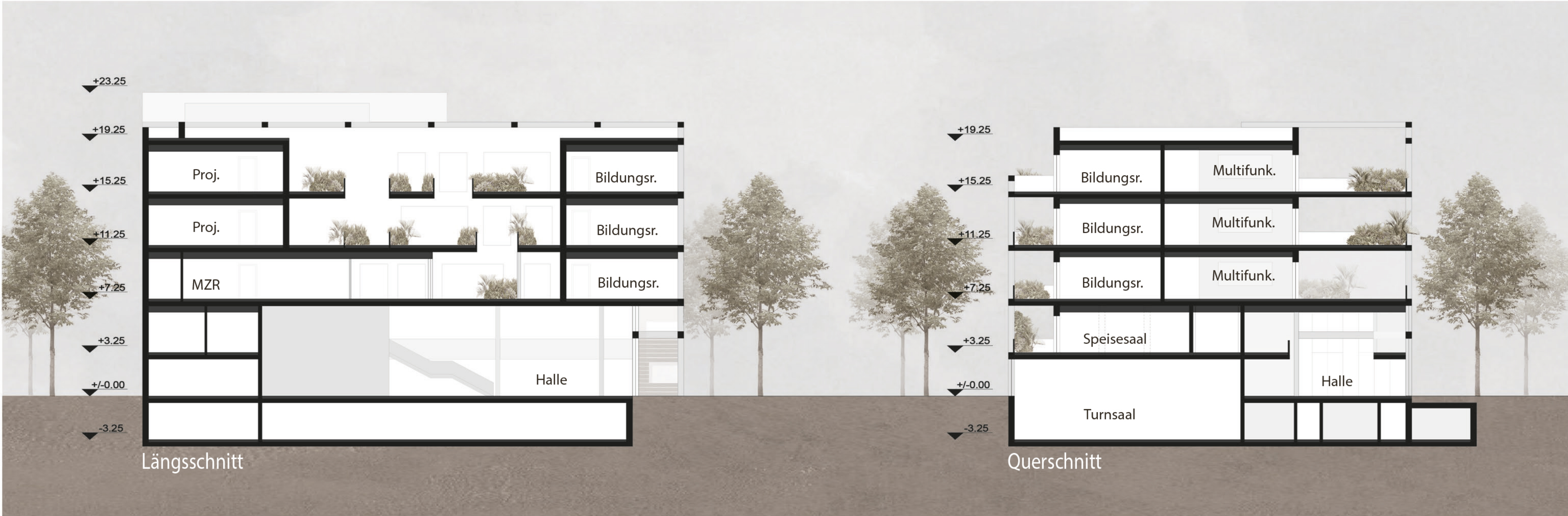
Systemcrosschnitt M:1.500
