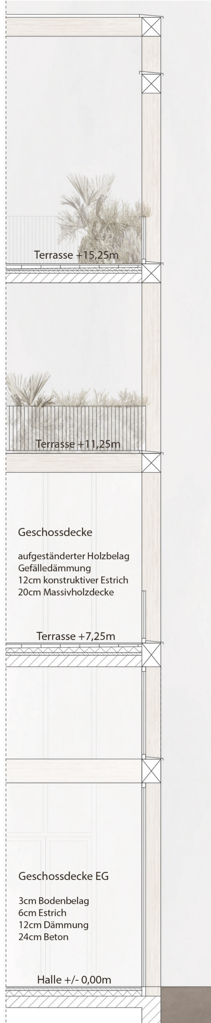
Fassadenschnitt M:1.50
